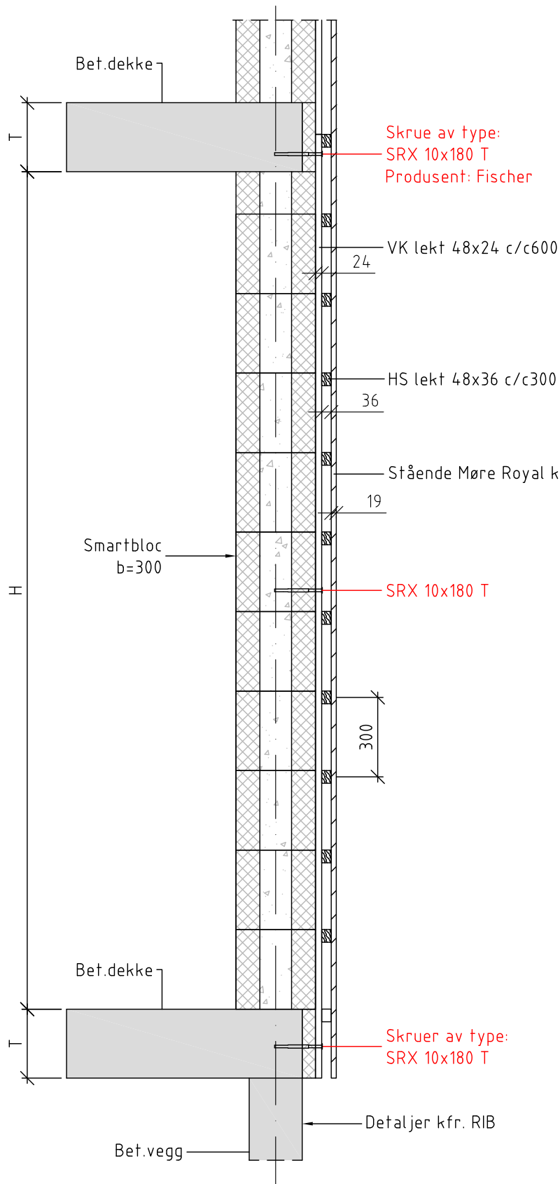
Generell detalj for festing av VK lekter M=1:20
